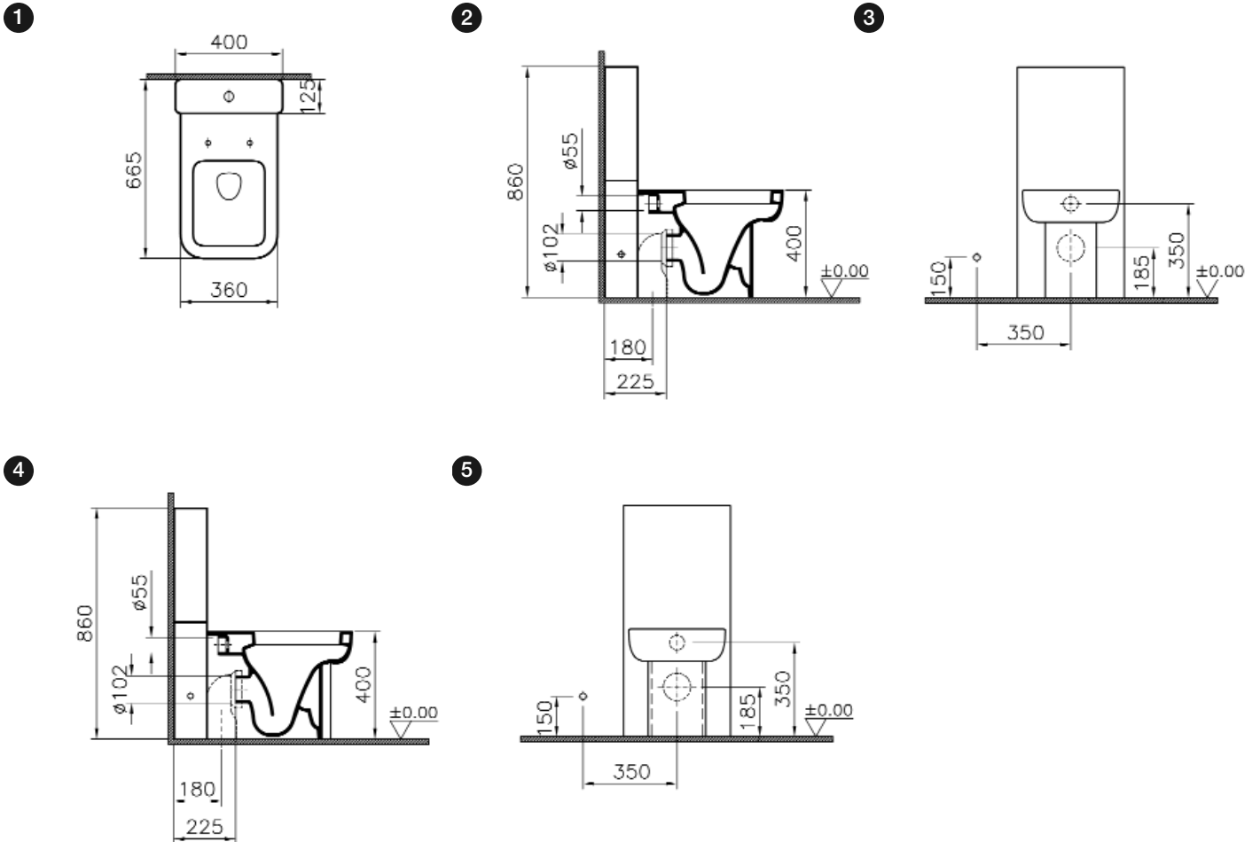
5354+Floor Standing WC Pan & Monoblock Cistern & WC Cover / Yerden Klozet & Kolon Rezervuar & Ayak / Stand-Tiefspül WC & Monoblock Spülkasten & WC Verkleidung
