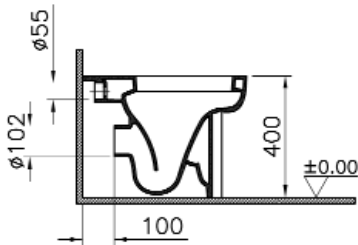
5354+Floor Standing WC Pan & WC Cover / Yerden Klozet & Ayak / Stand-Tiefspül WC & WC Verkleidung
